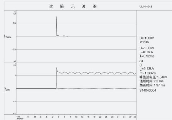
1000V UL In20A/40.3kA
