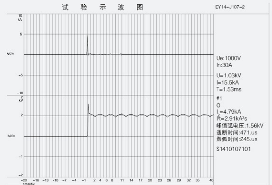
1000V In30A/15.5kA
