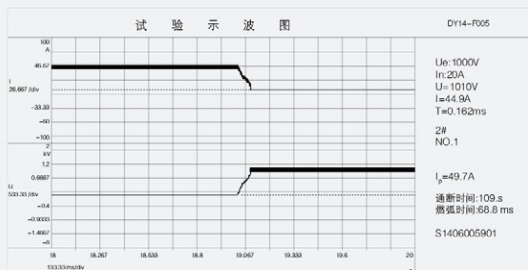
1000V UL In20A/40.3kA 预期电流示波图
