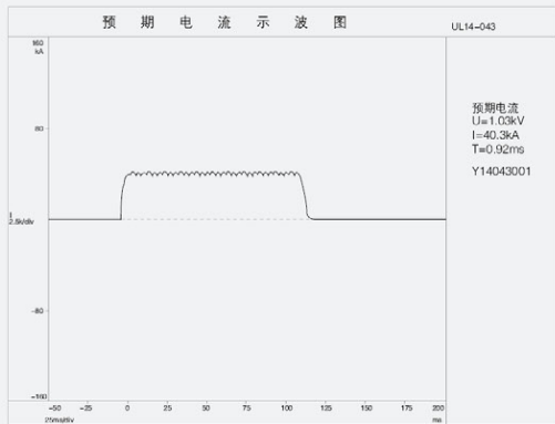
1000V UL In20A/40.3kA 预期电流示波图
