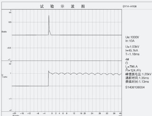
1000V In10A/45.1kA
