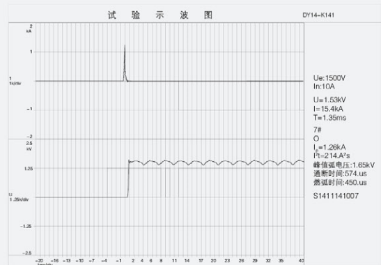
1500V In10A/15.4kA
