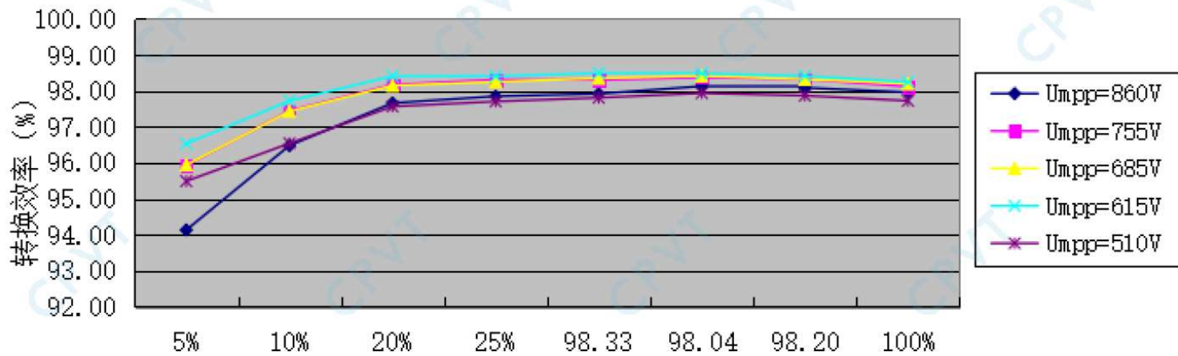
不同直流輸入電壓下的轉換效率 (GW50KS-MT)
