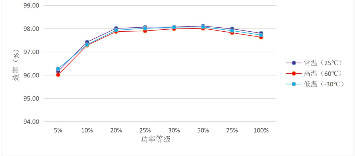
效率曲线 GW60KS-MT
