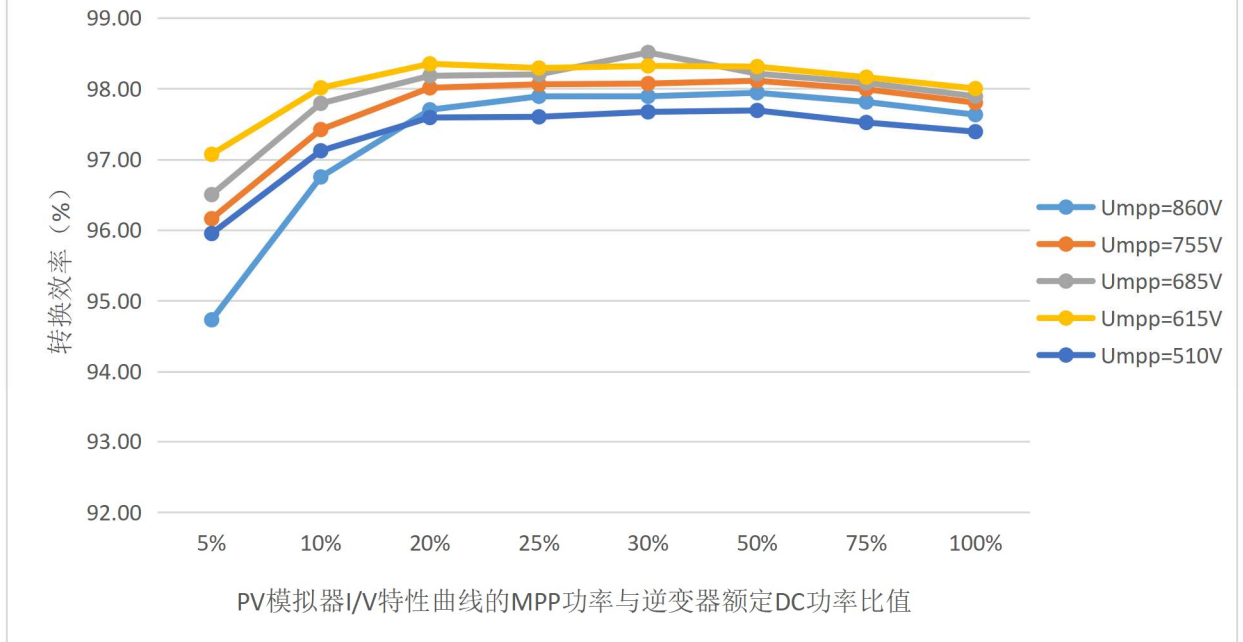
不同直流输入电压下的转换效率 GW60KS-MT
